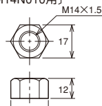
補助ストッパ用ナット SZZ (A2M14N010用)
