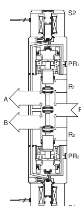
SR562-PN3 (ソレノイドS1、S2とも非通電)
