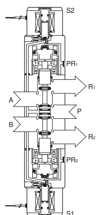
SR562-EN3 (ソレノイドS1、S2とも非通電)
