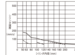
10H-2 負荷率50%
