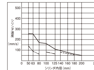
10H-2 負荷率0%
