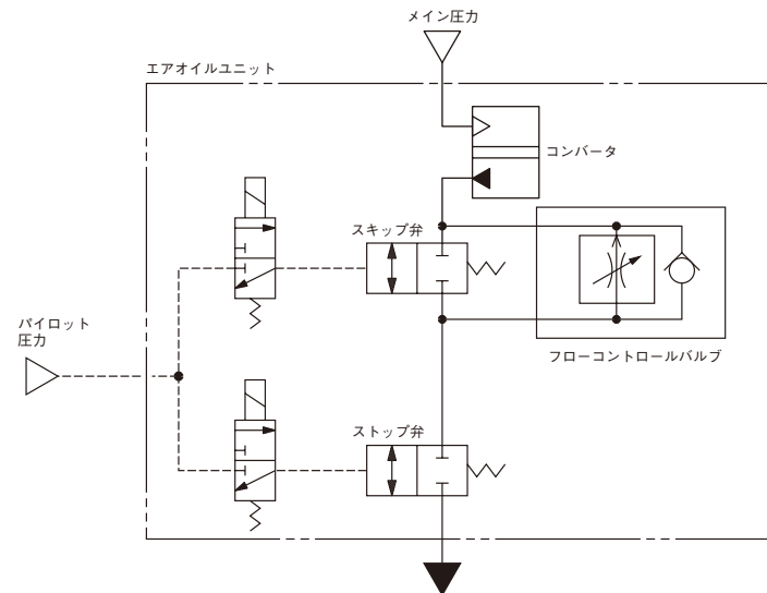
上図は、AHU2-※※※※※-FDAOの回路図です。
