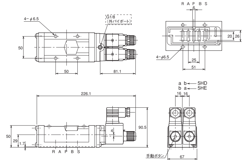
バルブ底面寸法
