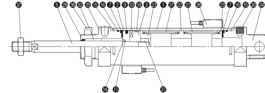
スプリングブッシュ(SH形)
