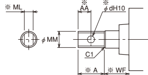
基準寸法表
