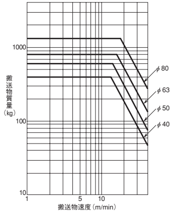
10G-2 SM- φ40 φ50 φ63 φ80-50st
