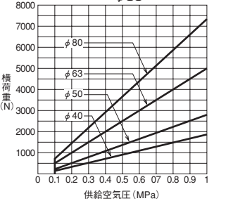
10G-2 SM- φ40 φ50 φ63 φ80-50st
