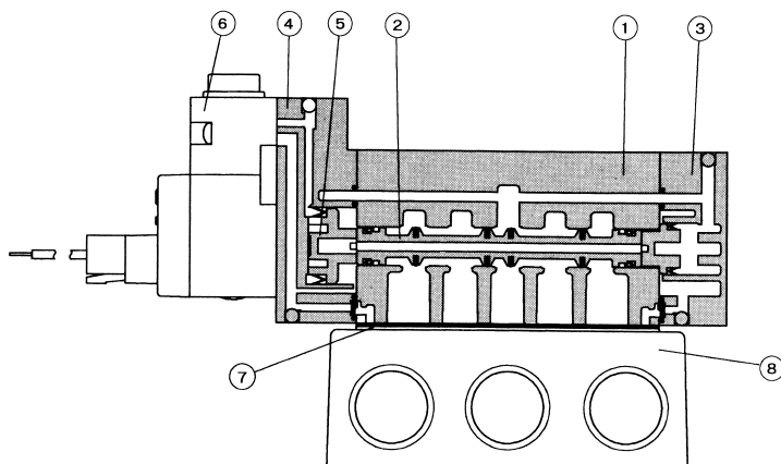
2位置シングル
