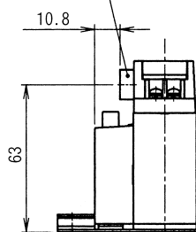
Dサブコネクタ横取出し
