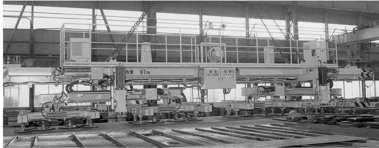
16ton鋼板搬送用バキューホースト
