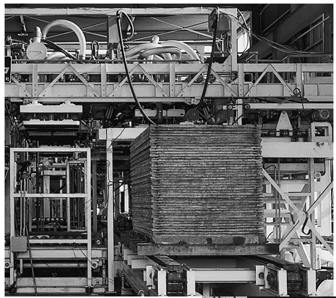
ボード搬送装置
