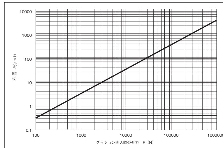
100H-2のクッション突入時の外力-エネルギー変換図
