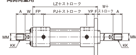
両ロッド形(φ32~φ250/B・Cロッド) 両側荷重用
