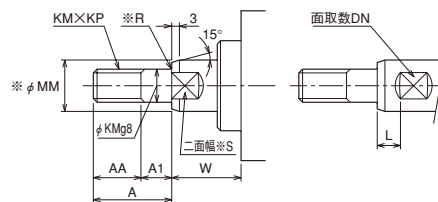
基準寸法表
