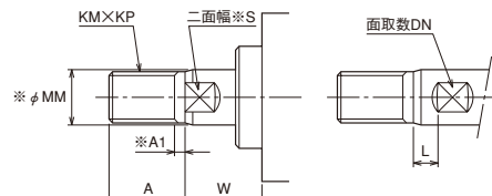
基準寸法表
