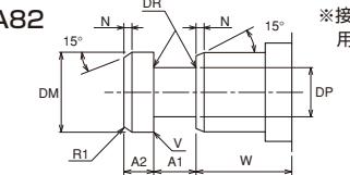
基準寸法表
