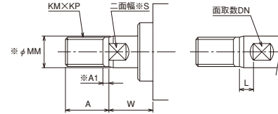
基準寸法表
