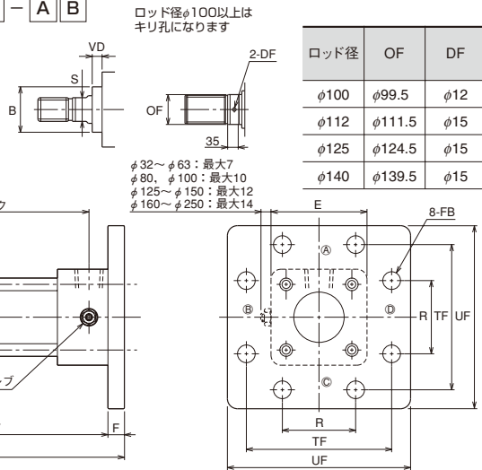
両ロッド形(φ32~φ250/B・Cロッド) 両側荷重用
