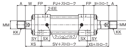
複動形両ロッド (B ロッド)
