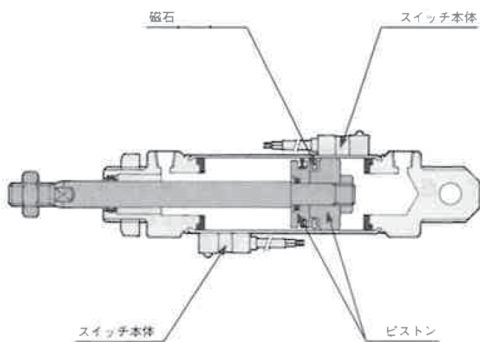
上図は、10Z-3Rの内部構造図です。
