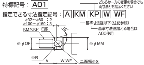
基準寸法表 (= 160H-1 標準寸法)
