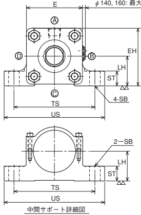
中間サポート詳細図
