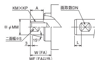
基準寸法表
