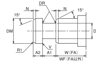
基準寸法表
