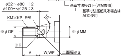
基準寸法表 (= 100H-2標準寸法)
