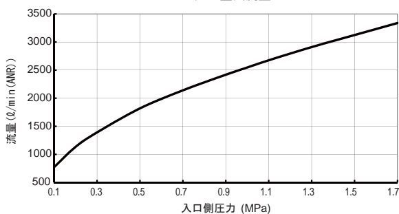
P33処理空気流量
