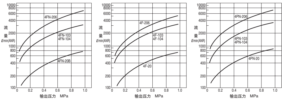
流量特性图
