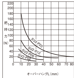
単動形/SV2-P※
