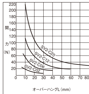
単動形/SV2-C※
