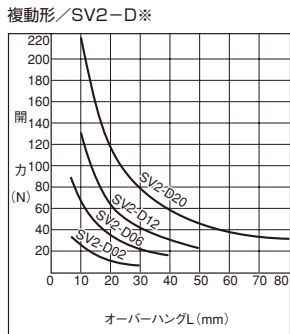
理論開力(供給圧力: 0.5MPa時)
