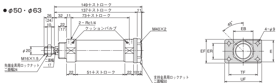
寸法表
