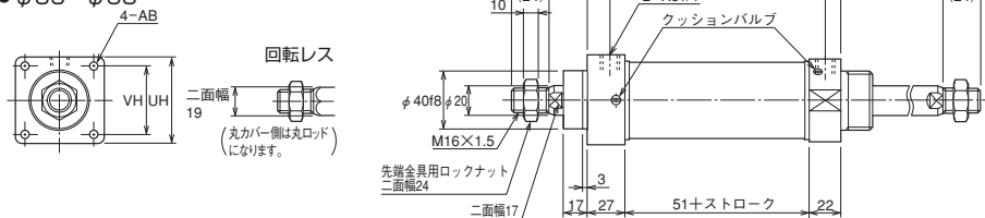
寸法表
