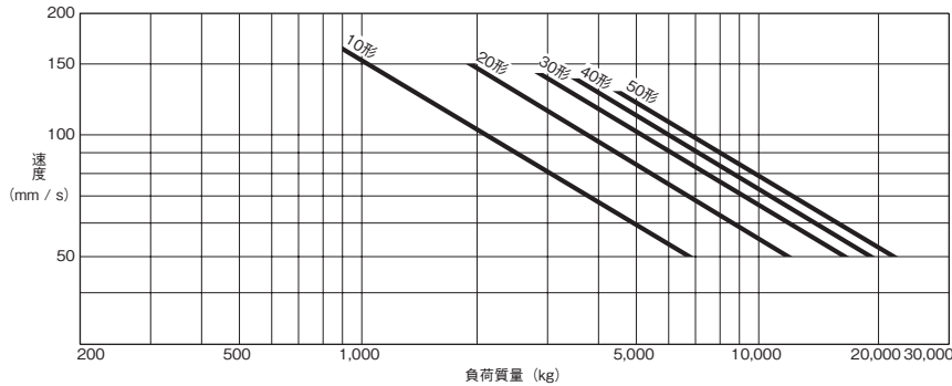
負荷質量－速度線図(水平送りの場合)
