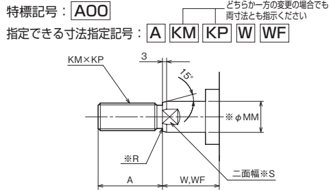
基準寸法表
