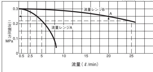
流量特性図 (流体: 水道水)
